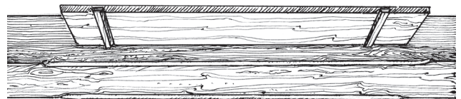
Іл. 33. Одинарна полиця, вмонтована на кілках понад фасадними вікнами у хаті поч. XX ст., с. Городниці (Гор. ІФ.). Рисунок В. Сивака
