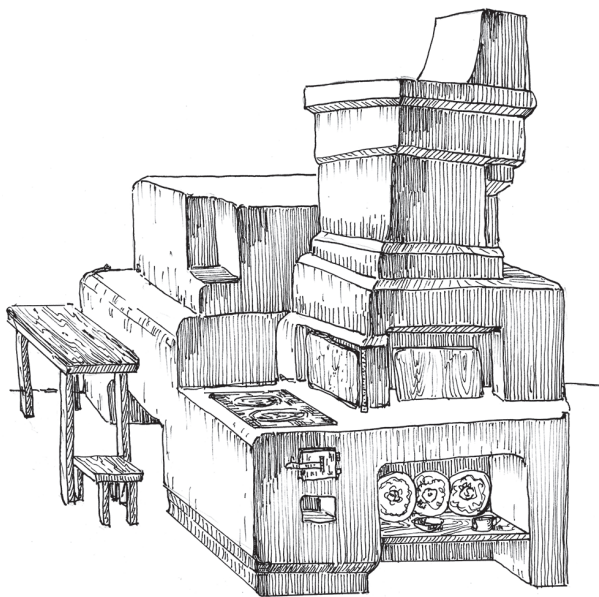
Іл. 36. Одинарна полиця, вмонтована під підпиччям у хаті поч. XX ст., с. Серафінці (Гор. ІФ.). Рисунок В. Сивака
