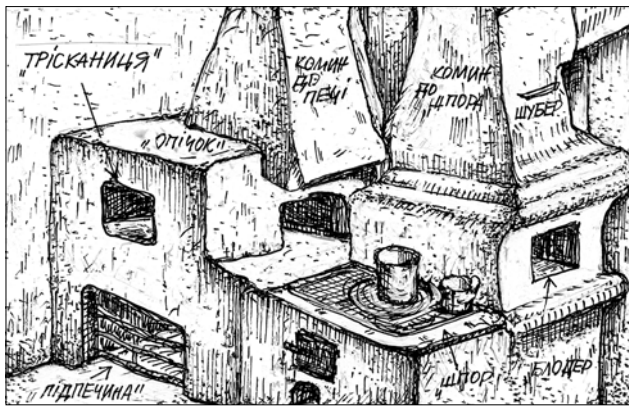
Іл. 3. «Трісканиця» — пічка, вимурувана в опічку печі, у якій сушили тріски для підпалу та скіпки для освітлення у хаті, збудованій у 1918 р, с. Луги Рахівського району Закарпатської області, Гуцульщина. Рис. В. Сивака
