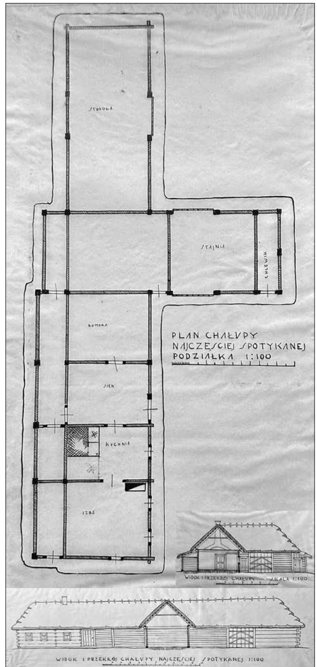
Іл. 16. Село Вербка. Найпоширеніша хата. Креслення Н. Боровської
