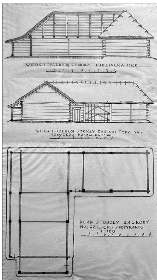
Іл. 20. Село Вербка. Г-подібні клуні. Креслення Н. Боровської
