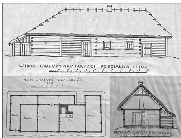
Іл. 13. Село Вербка. Найстаріша хата. Креслення Н. Боровської
