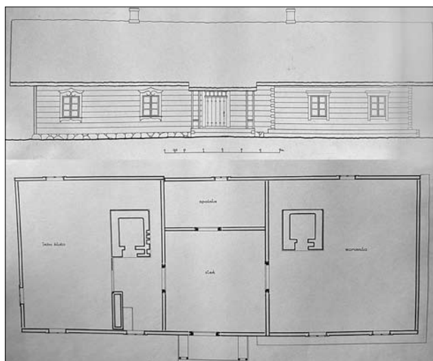
Іл. 14. Село Перешпа. Хата Сильвестра Жугара. Креслення з інвентаризаційної справи
