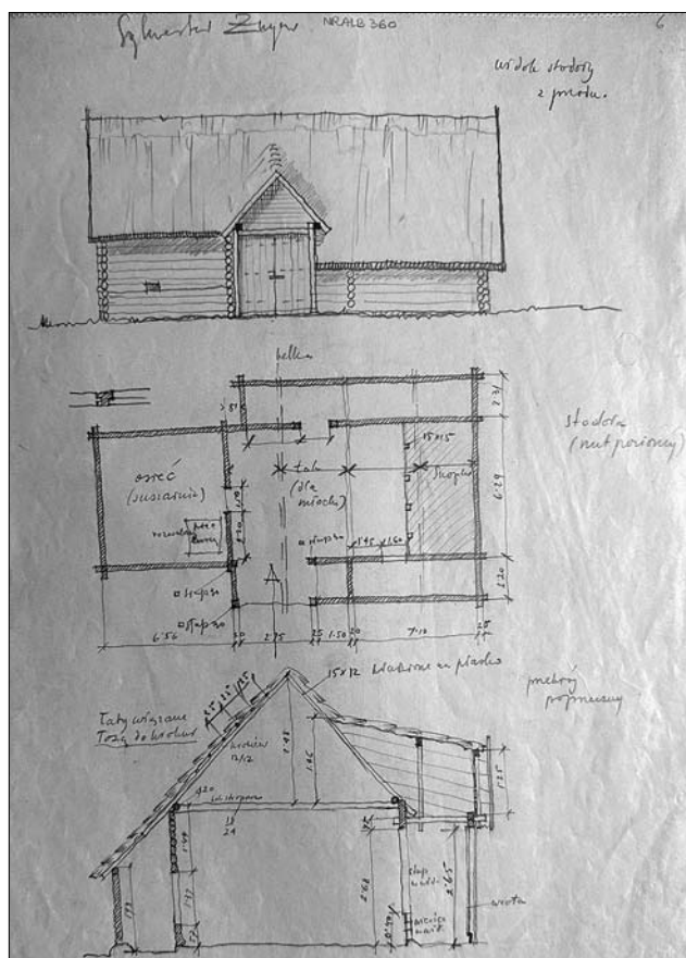
Іл. 21. Село Перешпа. Клуня Сильвестра Жугара, яка мстила осеть як частину клуні. Чернетка креслення з інвентаризаційної справи
