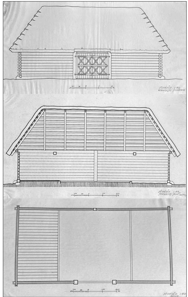
Іл. 19. Село Ланська. Клуня Герасима Олесюка. Креслення з інвентаризаційної справи
