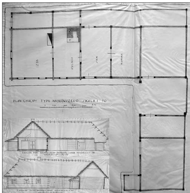
Іл. 15. Село Вербка. Найновіша хата. Креслення Н. Боровської
