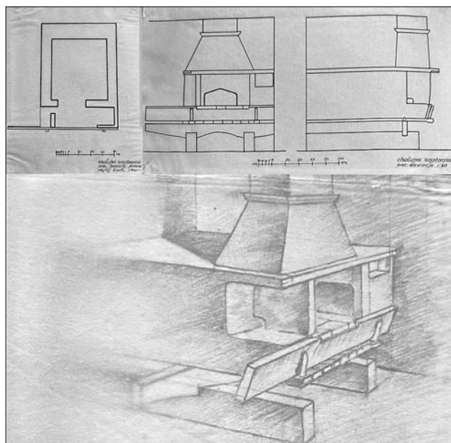
Іл. 12. Село Ланська. Під хати Владислава Чуля. Креслення та малюнок з інвентаризаційної справи
