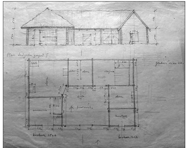
Іл. 7. Село Перешпа. Підварок Сильвестра Жугара. Чернетка креслення з інвентаризаційної справи
