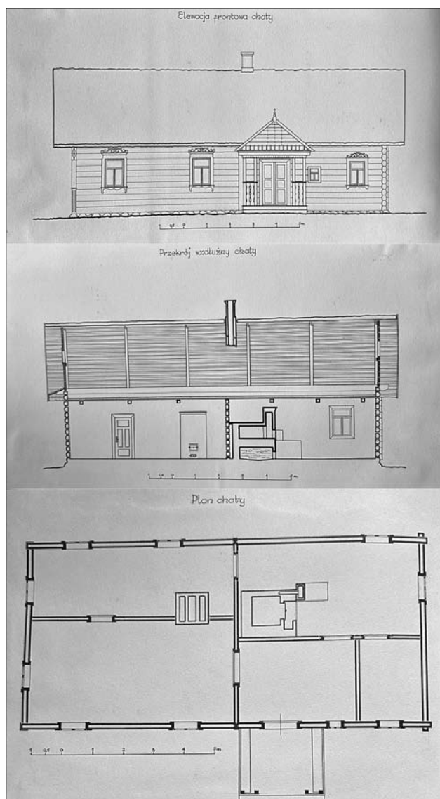
Іл. 18. Село Перешпа. Хата Фелікса Шипера. Креслення з інвентаризаційної справи
