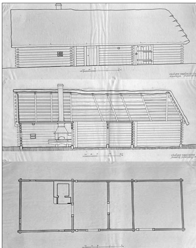
Іл. 11. Село Ланська. Хата Владислава Чуля. Креслення з інвентаризаційної справи
