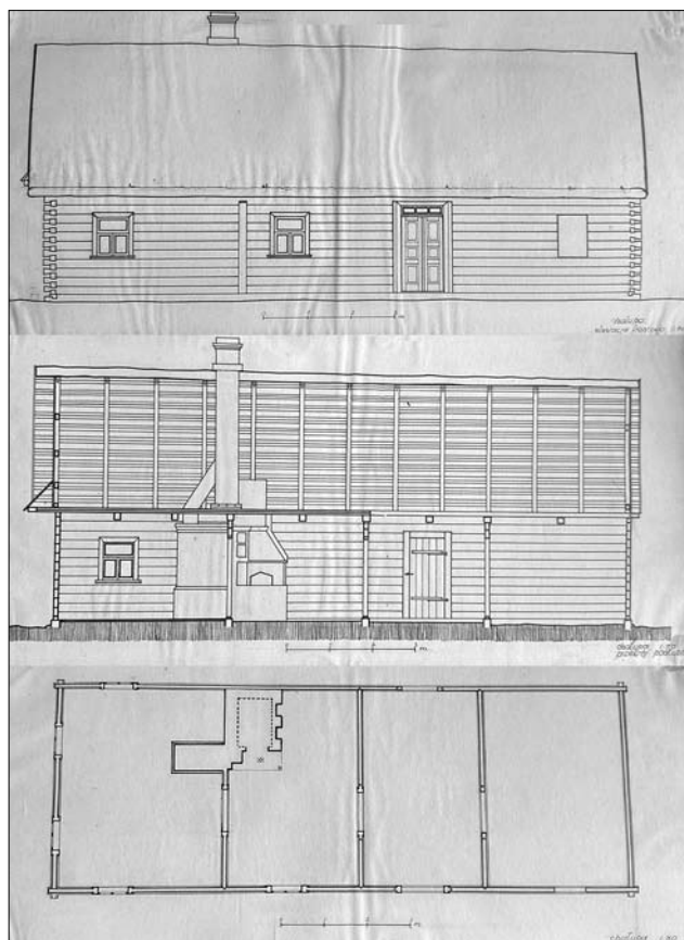
Іл. 17. Село Ланська. Хата Герасима Олесюка. Креслення з інвентаризаційної справи
