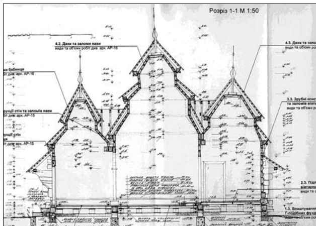
Іл. 13. Поздовжній розріз церкви. Архітектор М. Гайда
