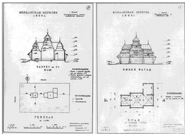
Іл. 9. Обміри церкви 1961 р. В. Корнєєвої та І. Макушенка. Архів інституту Укрзахідпроектреставрація
