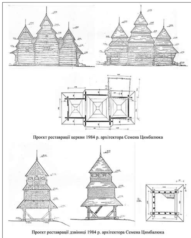
Іл. 10. Проєкт реставрації церкви та дзвіниці, 1984 р. Архітектор С. Цимбалюк
