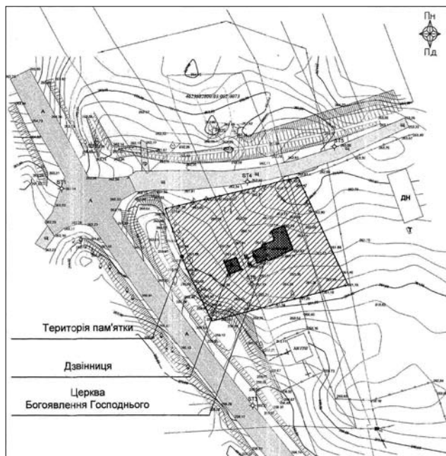
Іл. 1. Ситуаційний план. Арх. М. Гайда
