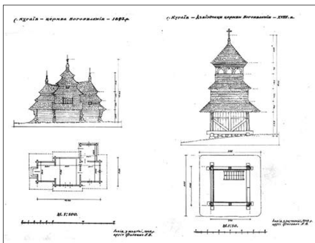
Іл. 8. Обміри церкви та дзвіниці 1948 р. архітектора Я. Фартуха-Філевича
