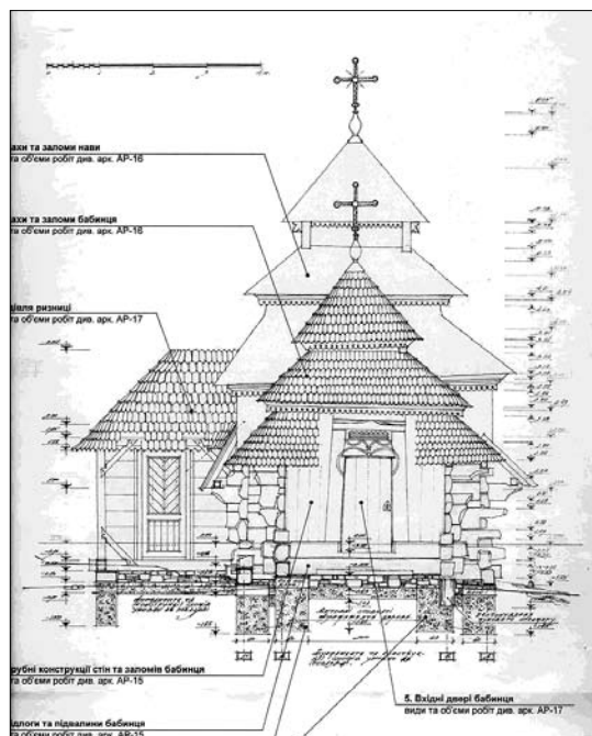
Іл. 11. Фасад церкви із заходу. Архітектор М. Гайда
